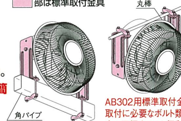
■AB302 設置例 (60Hz)
