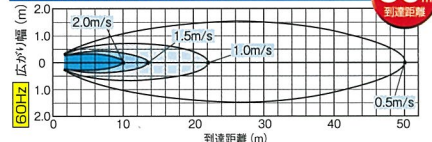
AB363NA/361NA 60Hz
