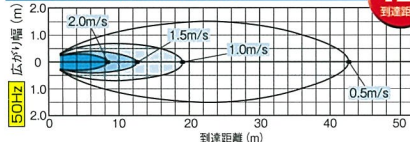
AB363NA/361NA 50Hz
