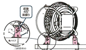
■AB36 設置例 (60Hz)
