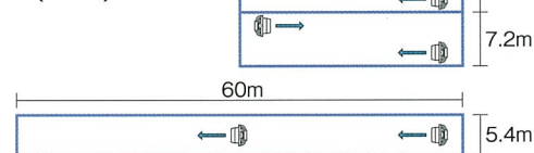
■AB27 設置例 (60Hz)
